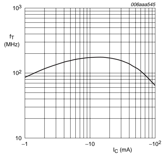
V_{CE} = -5\text{ V}; T_{amb} = 25^\circ\text{C}
